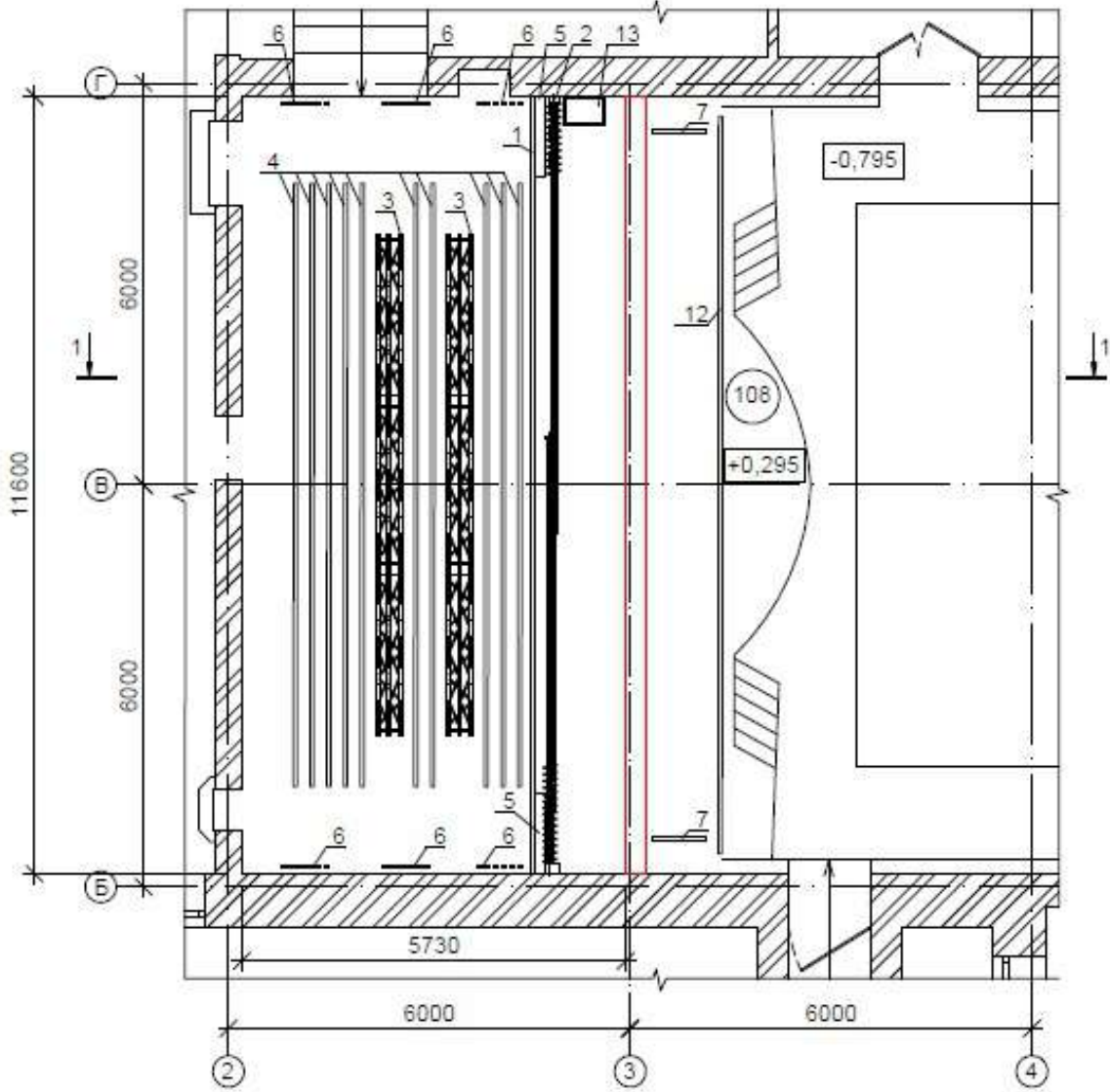
План 1 этажа
