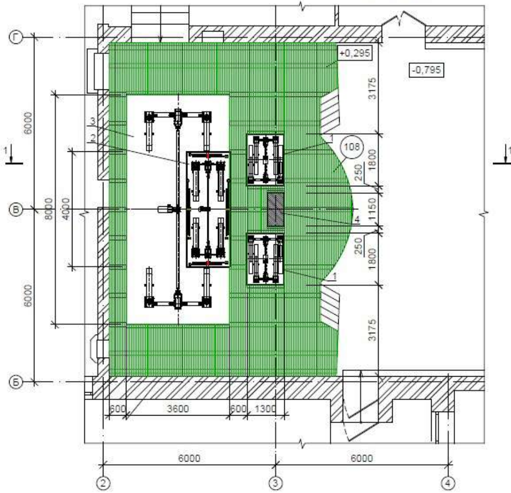
План 1 этажа
